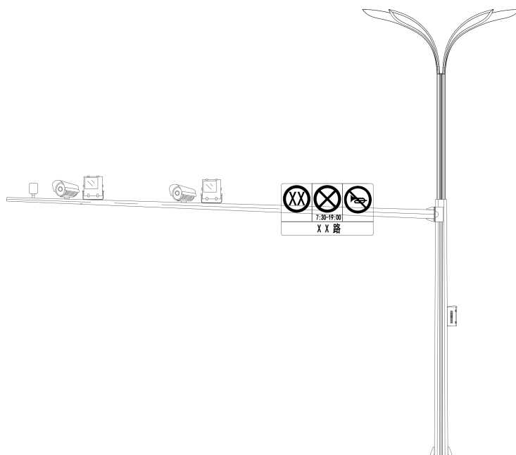
图 A-2 A2 类杆柱示意图
