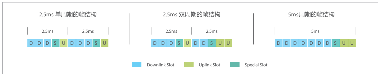
图 5G 主流帧结构
