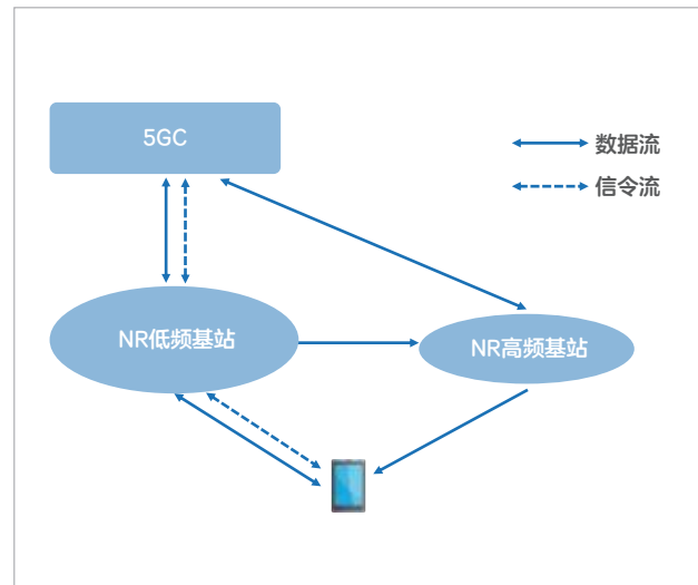
图 NN-DC 系统架构
