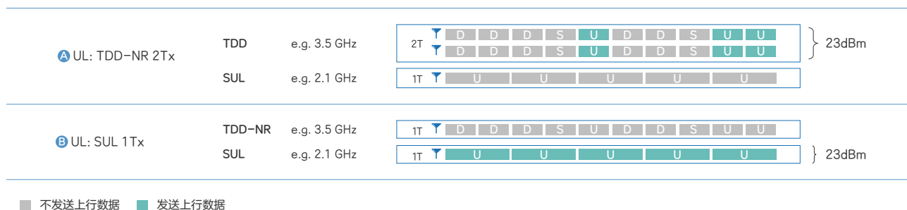
图 SUL 的终端上行工作模式
