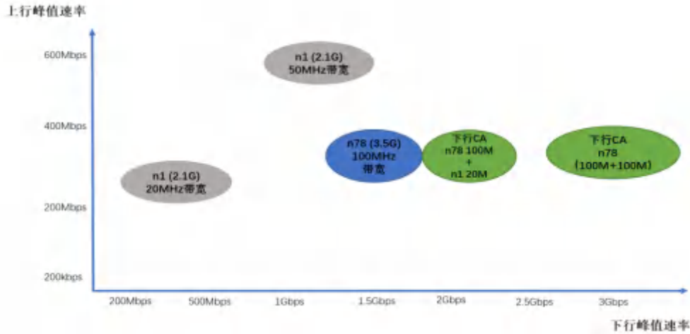
图 6 n1 以及 n78 频段上下行峰值速率 (SA 组网)
